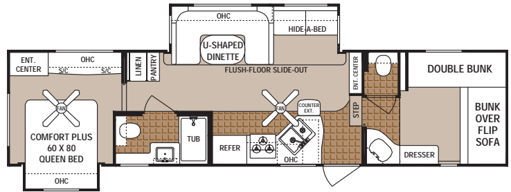
326QB-M5
