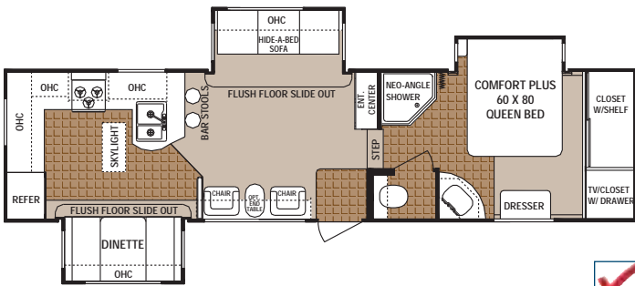
31RGSB-M5
